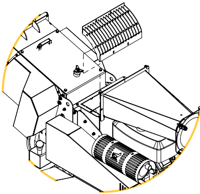
SIEB (OPTIONAL) Sieve (optional)
